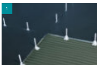
1 Umístěte nivelační základnu pod dlaždice cca 10 cm od každého konce.
