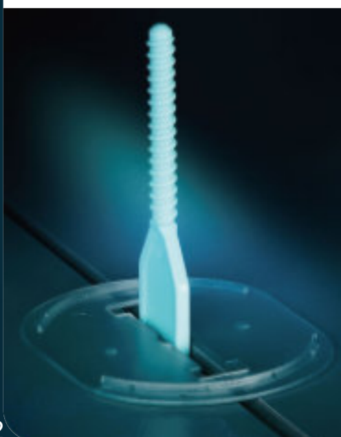
1 Umístěte nivelační základnu pod dlaždice cca 10 cm od každého konce.
