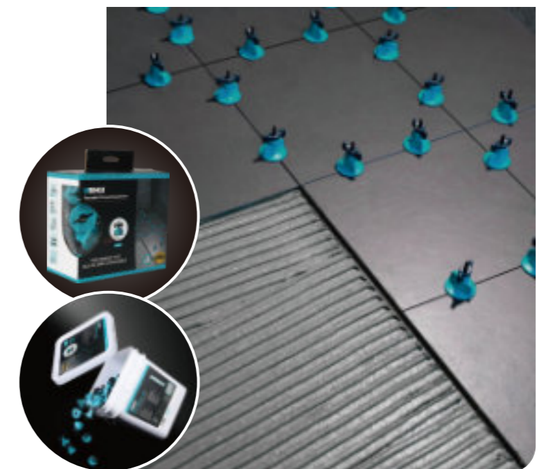
4 Pro opětovné použití otočte zpět o 90° do rovnoběžné polohy se spárou a vyjměte. (Pozn.: Vyjměte ihned po vyřízení – dle pokynů výrobce, nejpozději do 6 hodin.)
